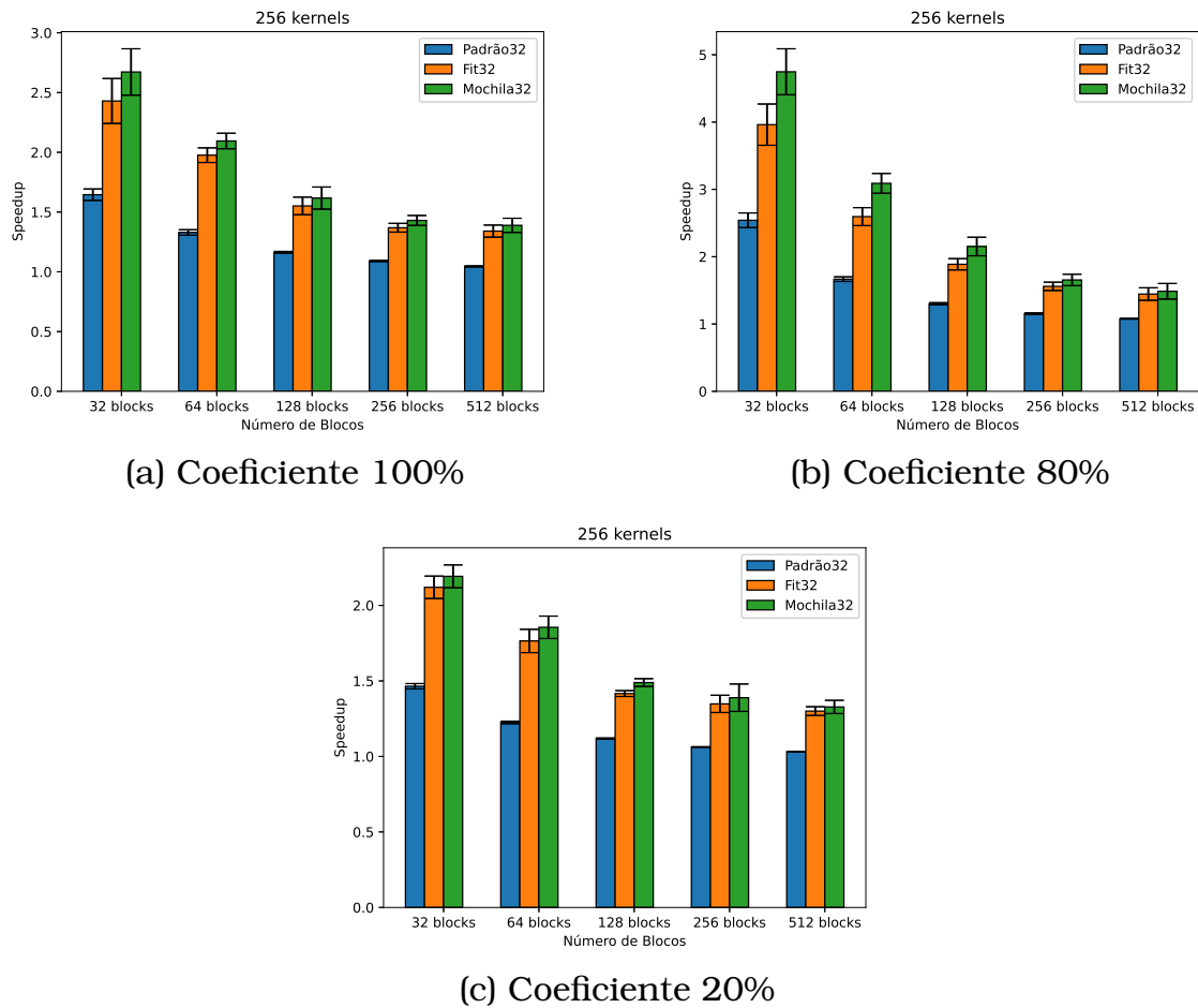
Figura 5.23: Proporção de melhora da média do tempo de resposta da execução paralela em relação ao tempo de resposta da execução sequencial para 256 kernels .
