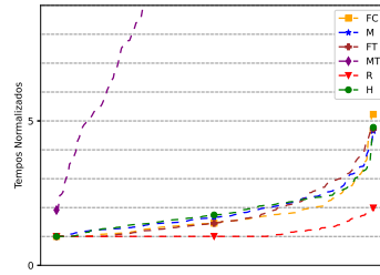
Figura 2.9: Curva-S dos cenários nos quais R é a estratégia com o menor impacto entre todas as GPUs.
