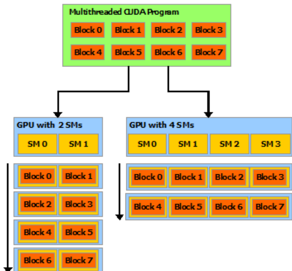
Figura 5.2: Os blocos de threads podem ter até 3 dimensões e são distribuídos entre os SMs da GPU.
