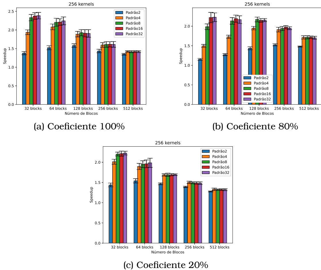
Figura 5.6: Impacto no tempo de duração da execução paralela em relação à execução sequencial para 256 kernels , usando a estratégia padrão.
