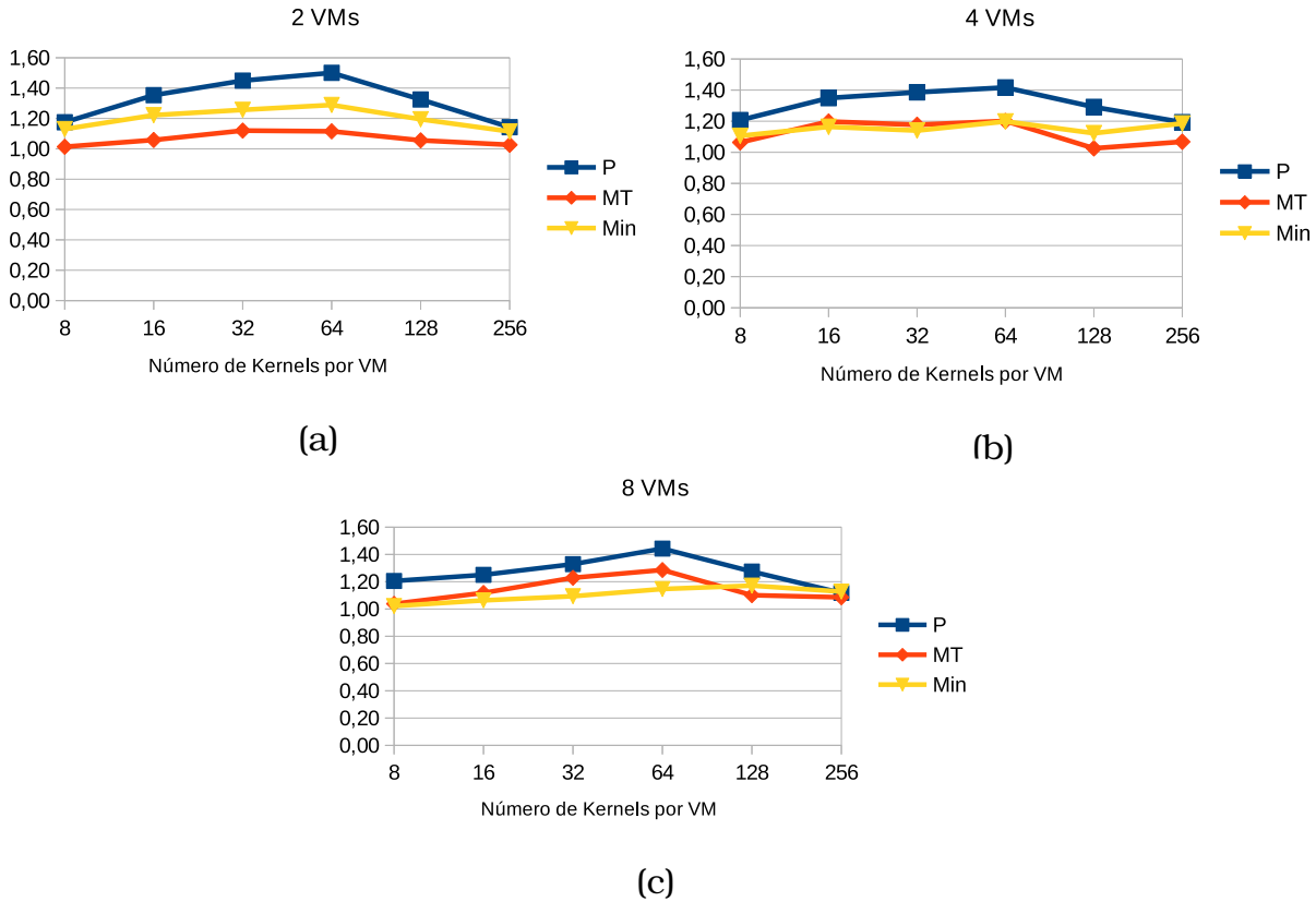
Figura 4.9: Speedup da implementação MinMT em relação às outras implementações em um ambiente homogêneo com: (a) 2 VMs, (b) 4 VMs e (c) 8 VMs.
