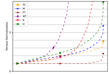
Figura 2.7: Curva-S dos cenários nos quais FT é a estratégia com o menor impacto entre todas as GPUs.
