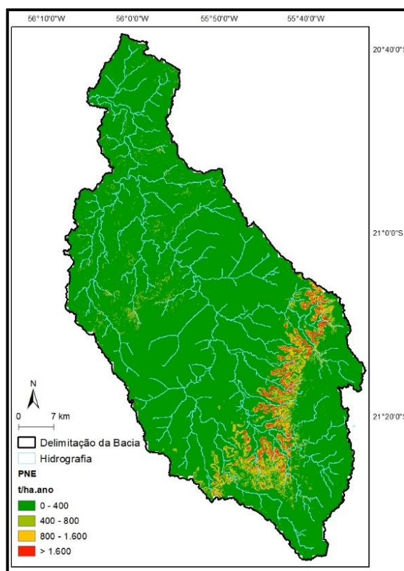
Figura 4 – Potencial Natural à Erosão Hídrica da bacia hidrográfica do Rio Nioaque – MS.
