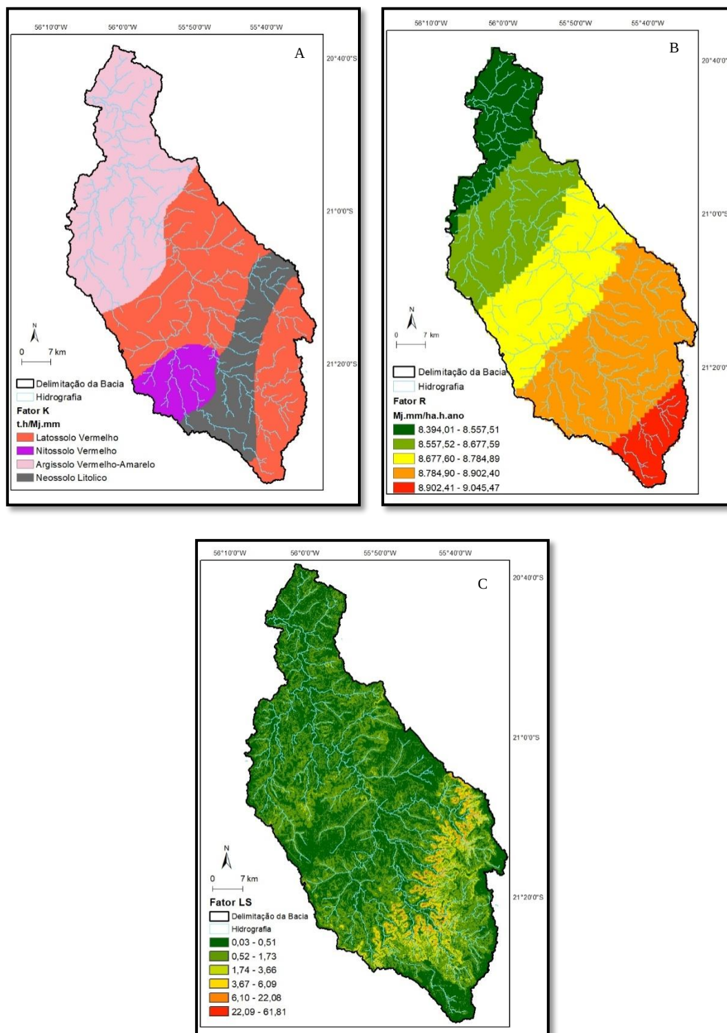
Figura 3 - Mapa do fator erodibilidade (A), fator erosividade (B), fator LS (C) da bacia hidrográfica do Rio Nioaque – MS.
