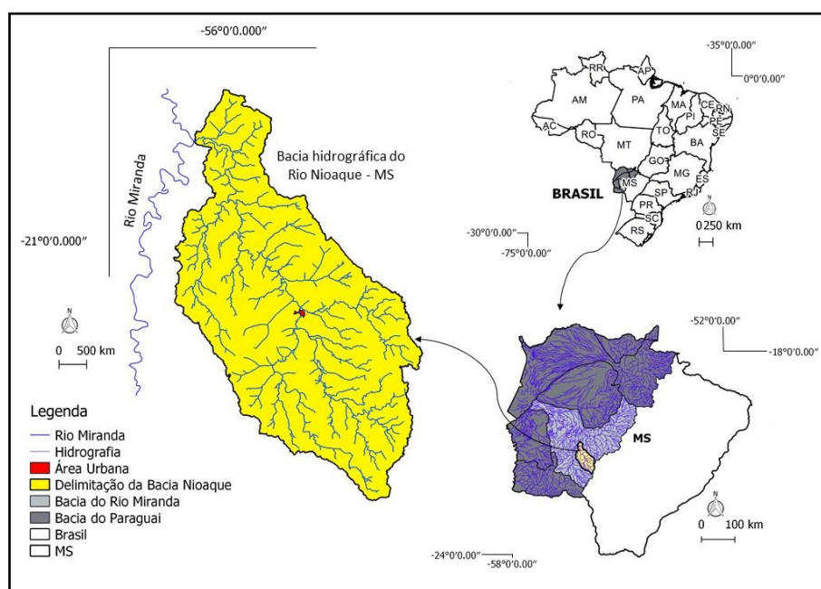
Figura 1 - Localização e delimitação da Bacia Nioaque – MS.
