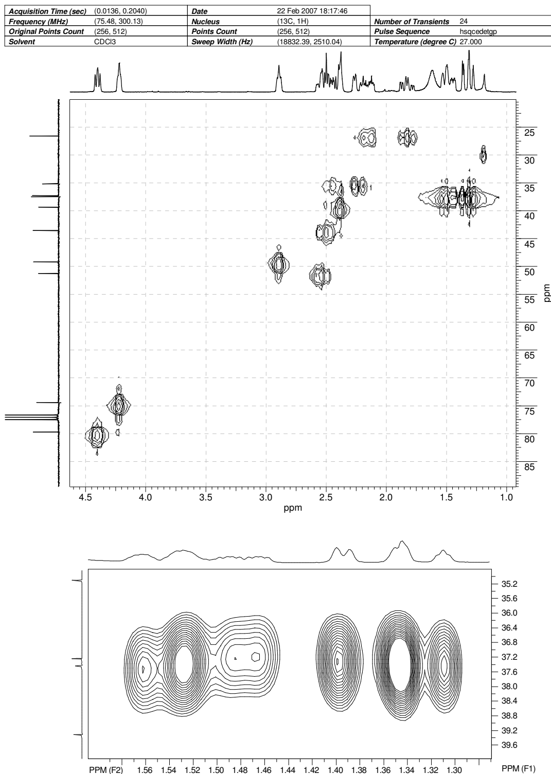
Figura 50: Espectro 2D (gHSQC; C/ H) do composto 15 .
