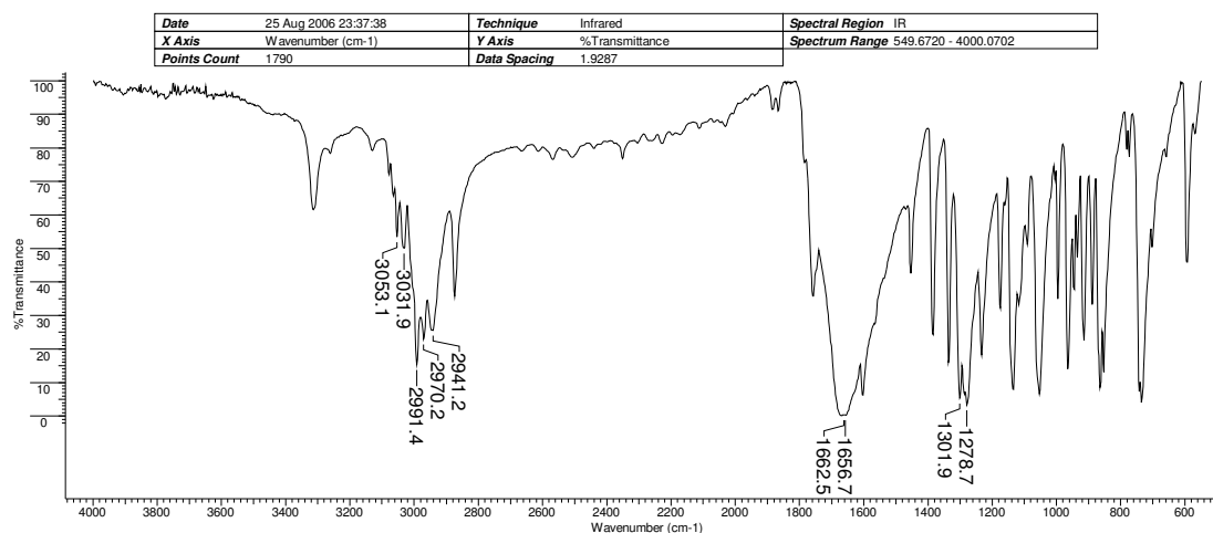
Figura 13: Espectro de IV do composto 7.
