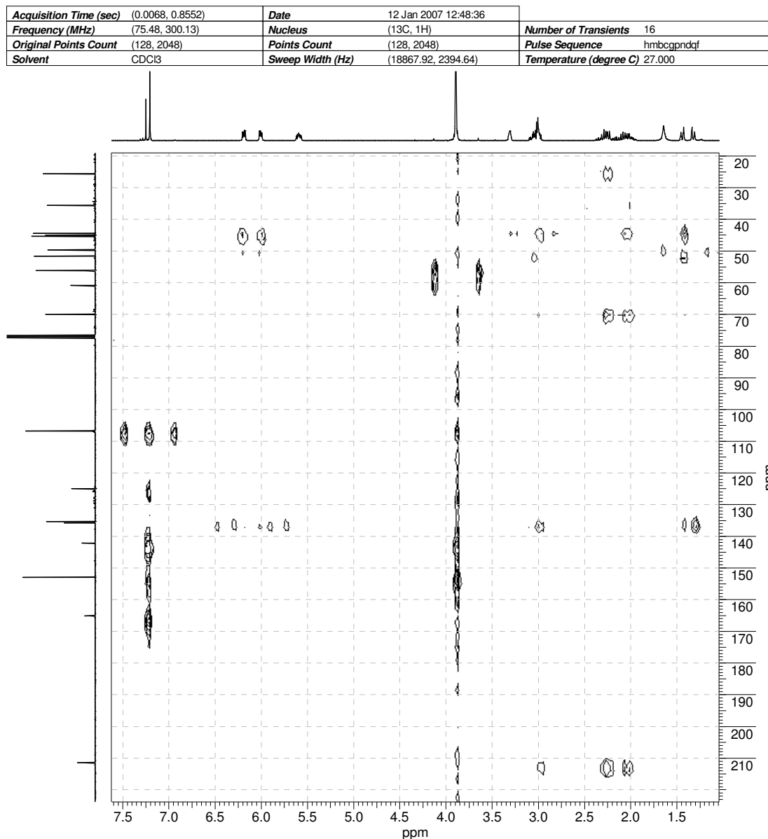
Figura 44: Espectro 2D (gHMBC; C/ H) do composto 34 .
