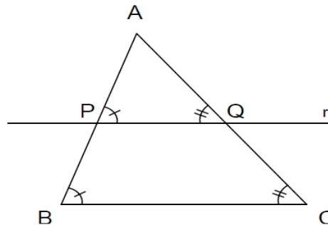
Figura 1.11: Teorema Fundamental da Semelhança.
