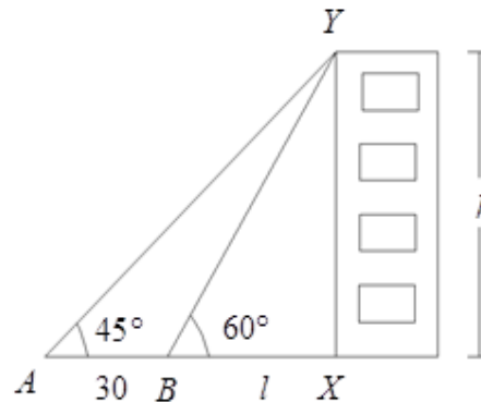
Figura 2.10: Aplicação das razões trigonométricas.
