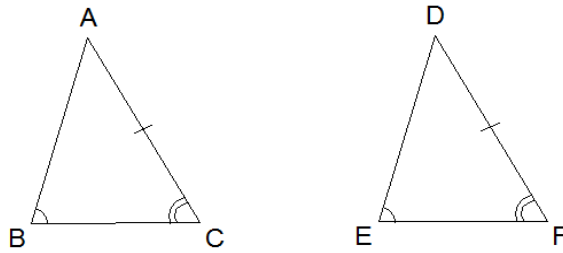
Figura 1.6: Congruência de triângulos \angle A A_0 .
