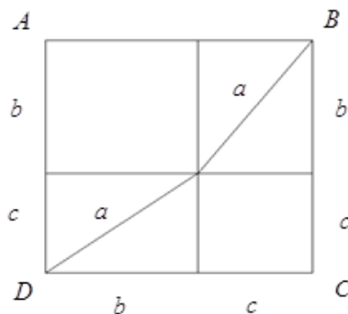
Figura 1.17: Demonstração do Teorema de Pitágoras.
