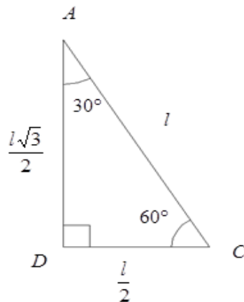
Figura 2.7: Dedução de seno, cosseno e tangente de 30^\circ e 60^\circ .
