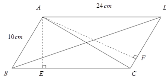
Figura 1.12: Paralelogramo ABCD .
