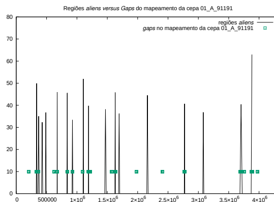
Figura 4.5: Posicionamento dos gaps da cepa 01_A_91191 em relação às 17 regiões aliens do genoma de referência.
