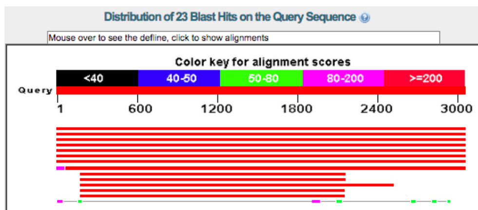
(a) Melhores alinhamentos.
