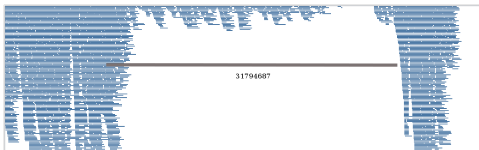
Figura B.3: Intervalo entre as bases 3.881.817 a 3.891.400 contido na região alien AR_{17} referente ao mapeamento da cepa 08_B_45-08B. O gene em destaque possui as coordenadas de 3.883.854 a 3.889.670 na referência.
