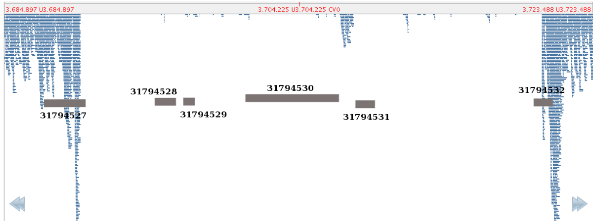
Figura 4.6: Trecho do mapeamento dos reads cepa 28_B_35 na região AR_{16} com indicação das posições relativas e PIDs dos genes anotados no genoma de referência.
