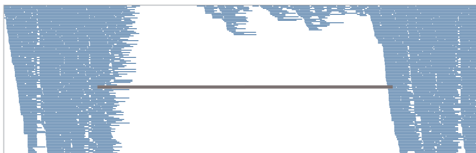
Figura B.4: Intervalo entre as bases 3.889.569 a 3.894.356 contido na região alien AR_{17} referente ao mapeamento da cepa 09_B_18-08C. O gene em destaque possui as coordenadas de 3.890.501 a 3.893.479 na referência.
