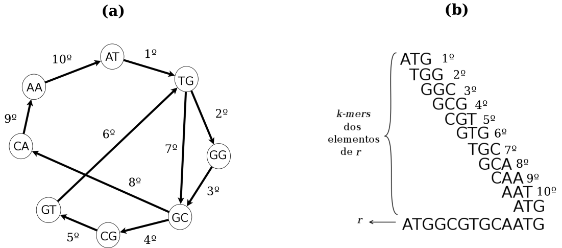
Figura 2.5: Grafo de Bruijn construído para os prefixos e sufixos de tamanho 2 presentes no 3-mers dos reads CGTGCAA , ATGGCGT , CAATGGC , GGCGTGC e TGCAATG .
