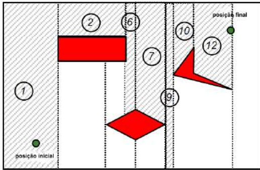
Figura 2.24: Aplicação do algoritmo para a escolha do caminho em DC. Fonte: Adaptado de CHAIMOWICZ, 2014, [9].
