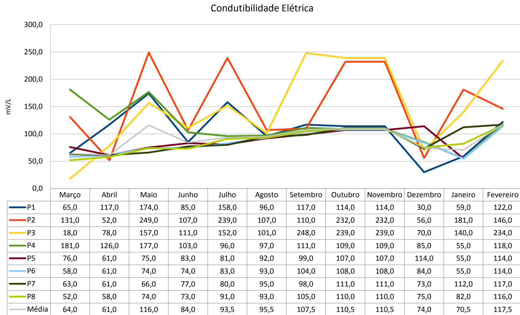
Figura 36.: Oscilação temporal da Condutividade Elétrica, na Lagoa Maior.
