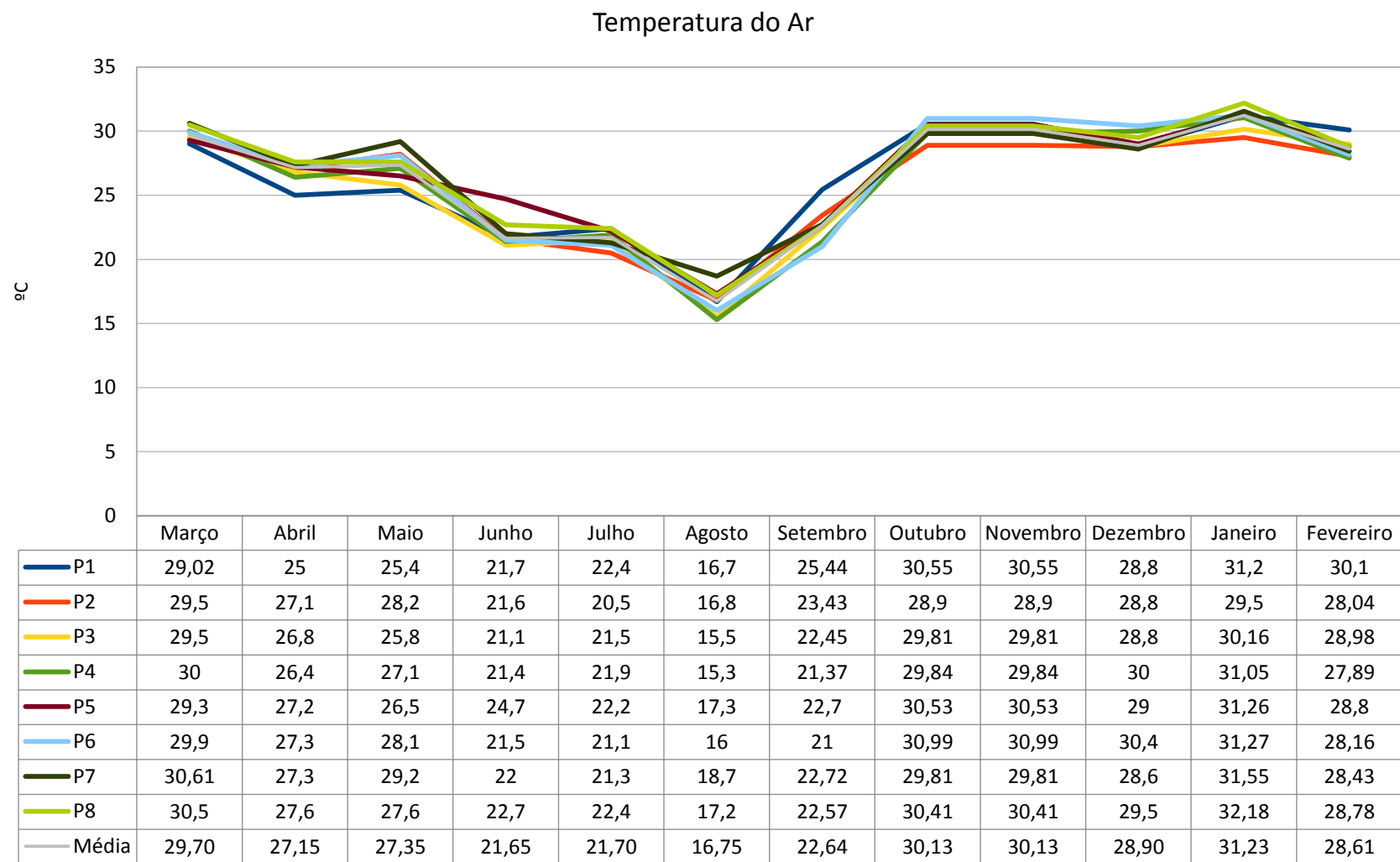
Figura 28: Temperatura do ar na Lagoa Maior.
