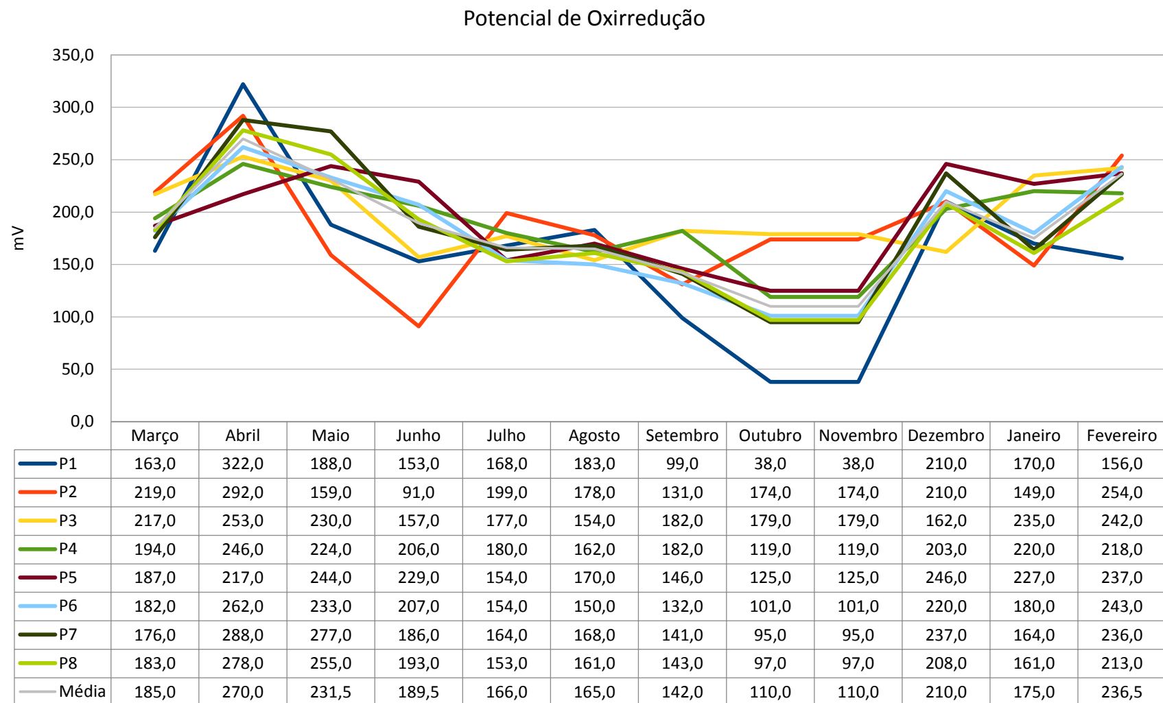
Figura 34: Análise do Potencial de Oxirredução na Lagoa Maior.
