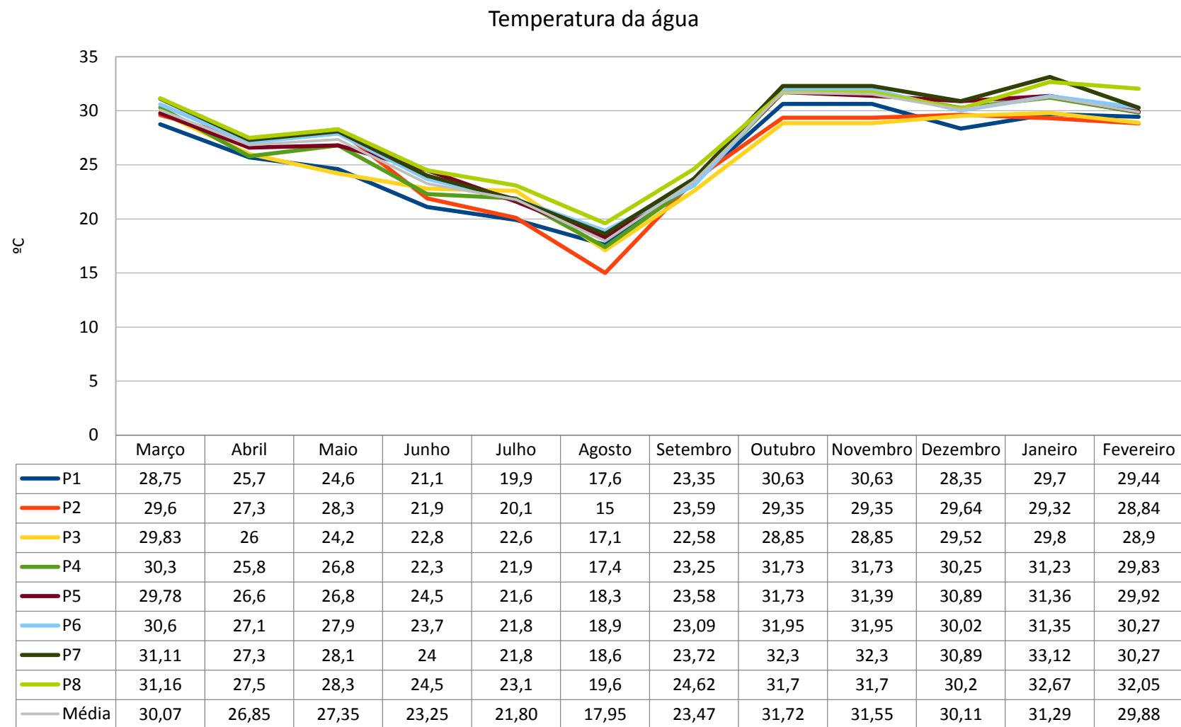
Figura 26: Temperatura da água na Lagoa Maior.
