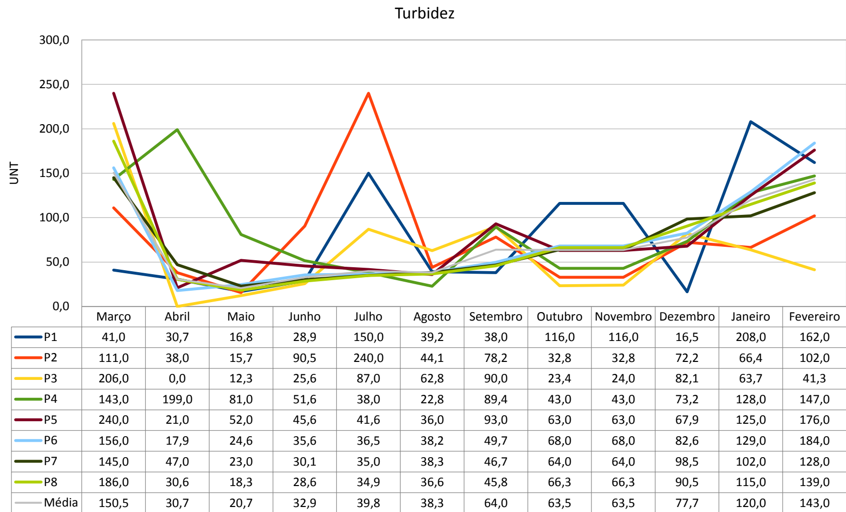
Figura 32: Valores de Turbidez na Lagoa Maior.
