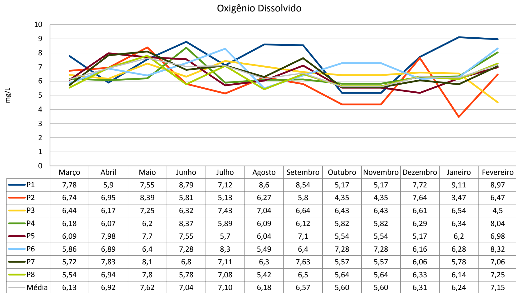
Figura 23: Concentração de oxigênio dissolvido na Lagoa Maior.
