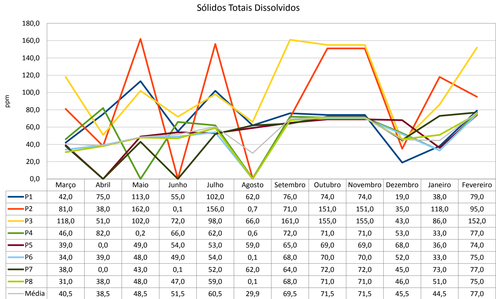
Figura 30: Concentração dos Sólidos Totais Dissolvidos na Lagoa Maior.
