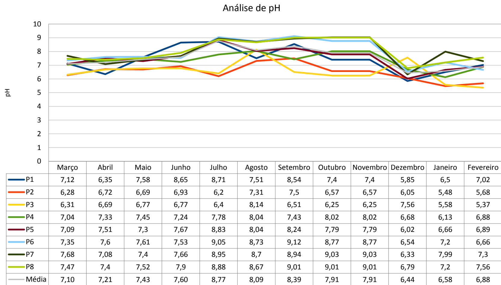
Figura 21: Análise de pH.
