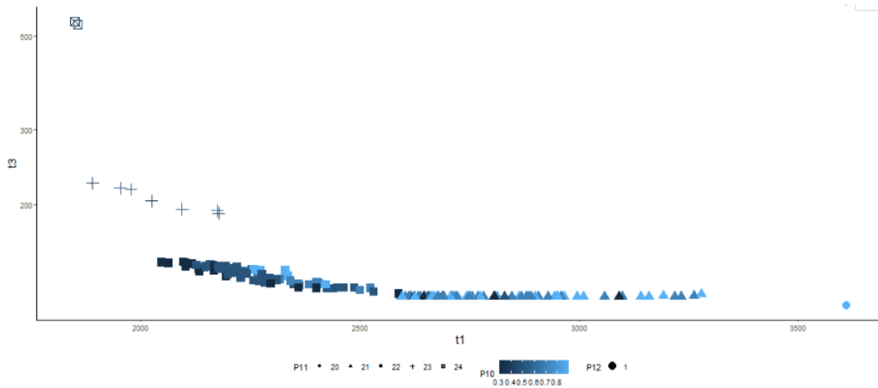
Figura 36 - Comparação dos objetivos t1 e t3 para os parâmetros P10 , P11 e P12 para Boa Vista
