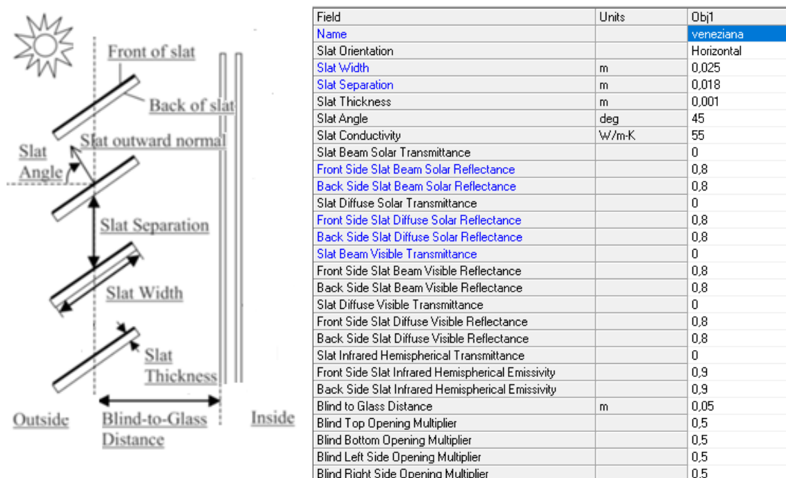
Figura 19 Detalhe da veneziana inserida com a janela
