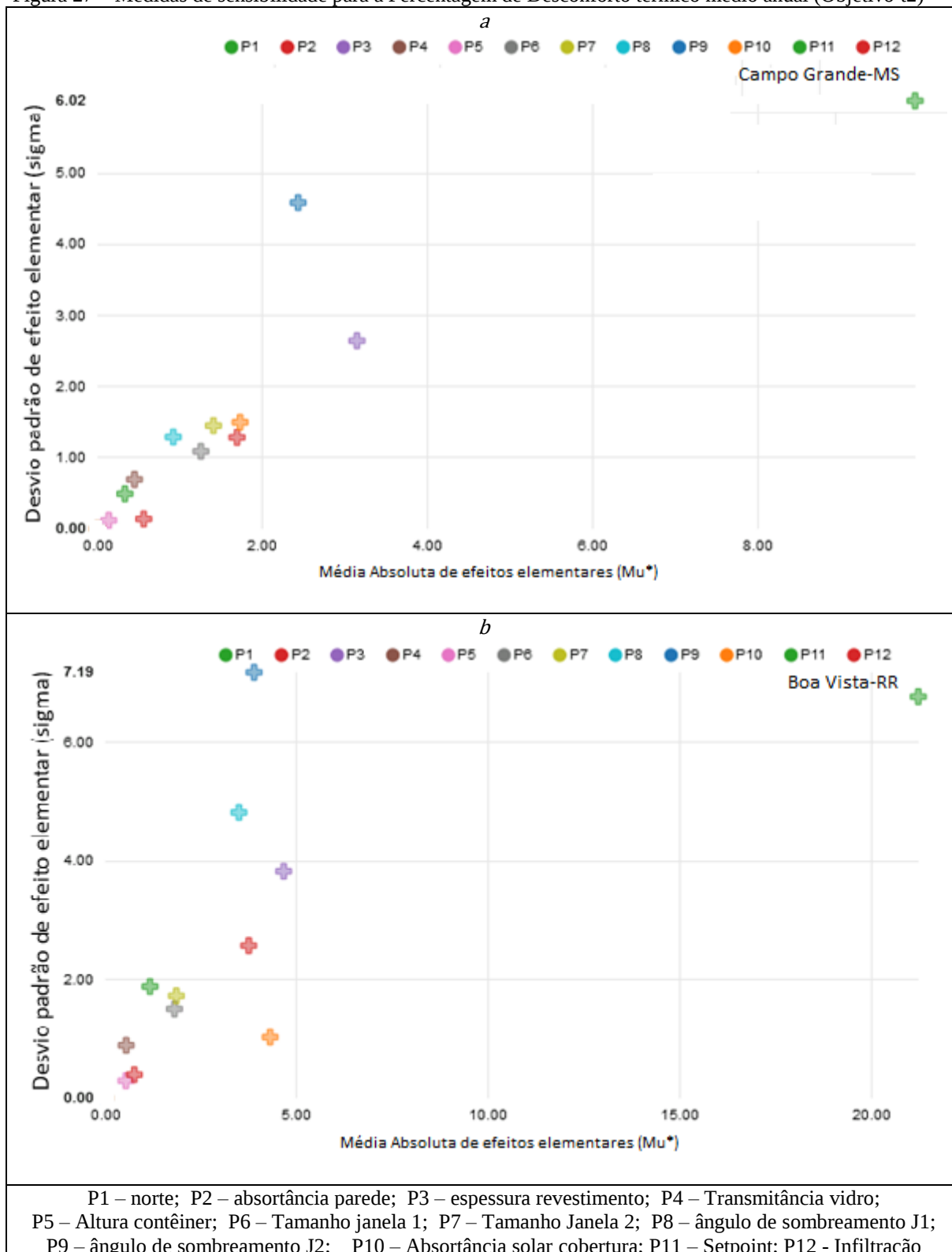
Figura 27 – Medidas de sensibilidade para a Percentagem de Desconforto térmico médio anual (Objetivo t2)
