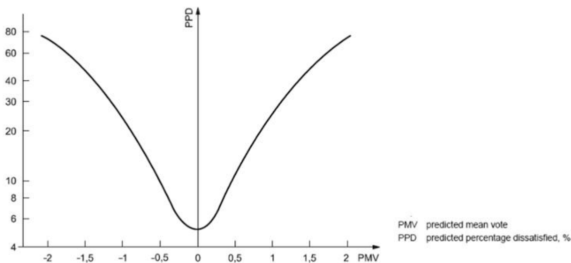
Figura 6 – Percentagem de pessoas insatisfeitas (PPD) em função do voto médio estimado (PMV)
