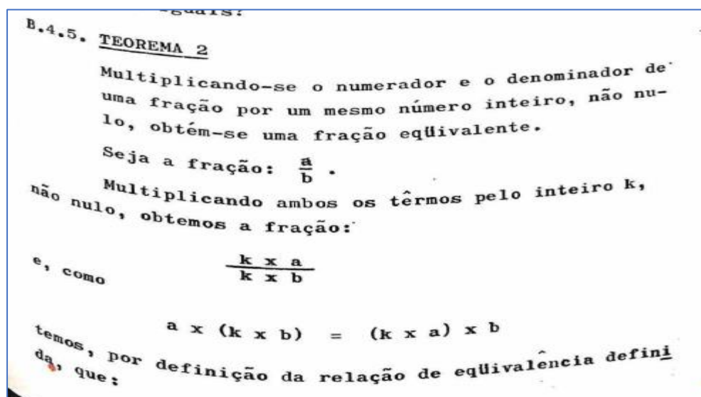
FIGURA 43 - Teorema
